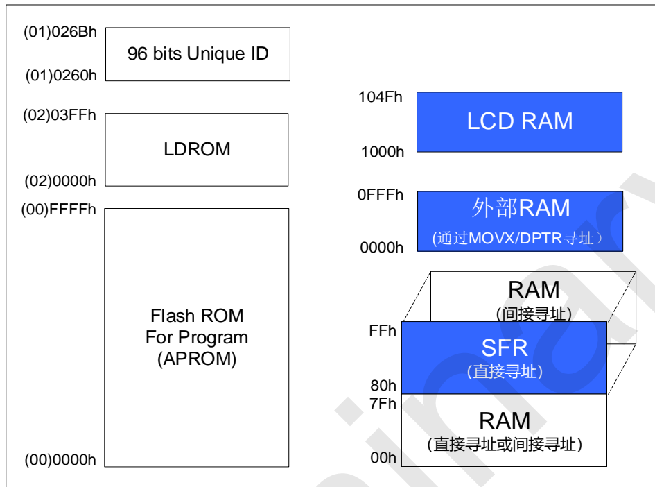
Flash ROM 和 SRAM 结构图
