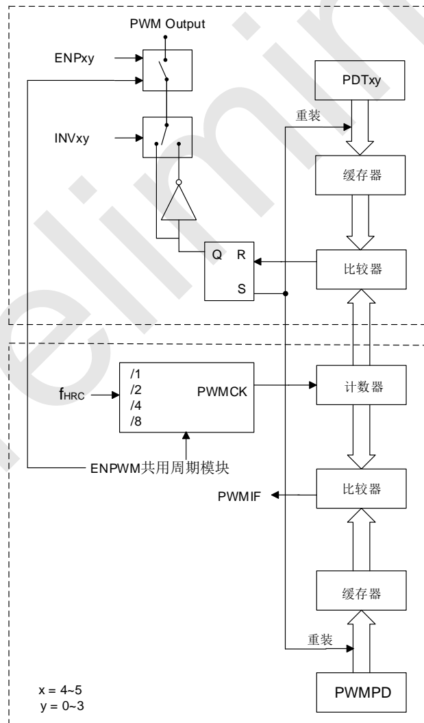
SC8FT67 PWM 结构框图
