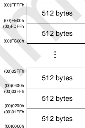
SC8FT67 64 Kbytes Flash ROM Sector 分区示意
