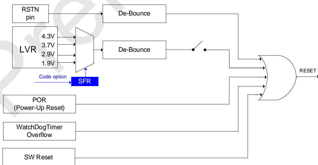
SC8FT67 复位电路图
