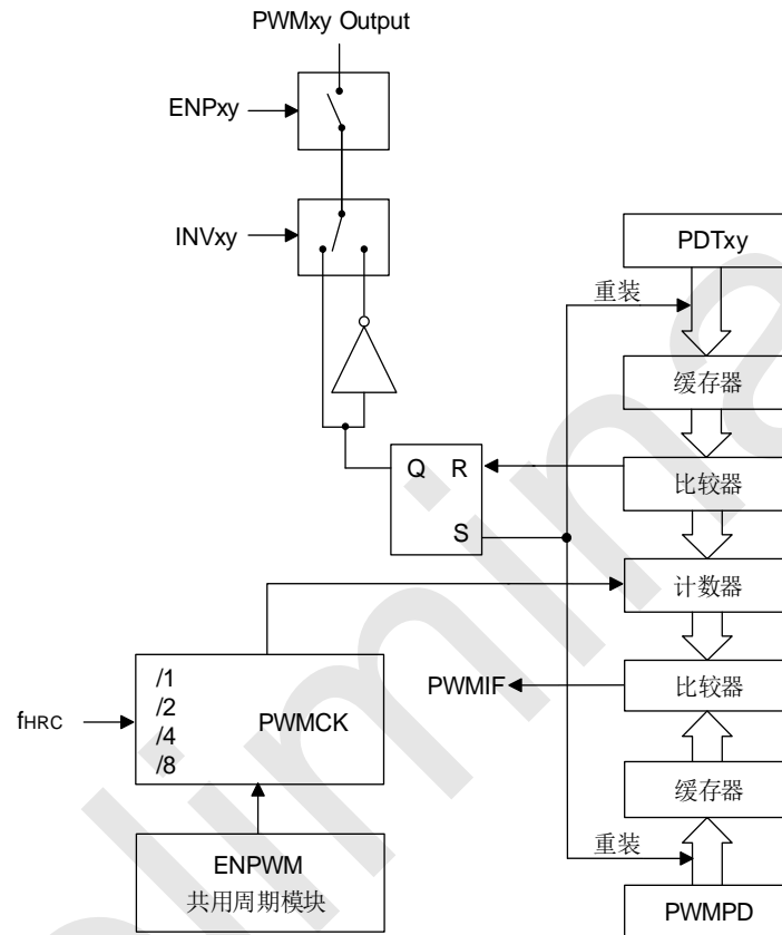
SC8FT67 PWM 独立模式框图
