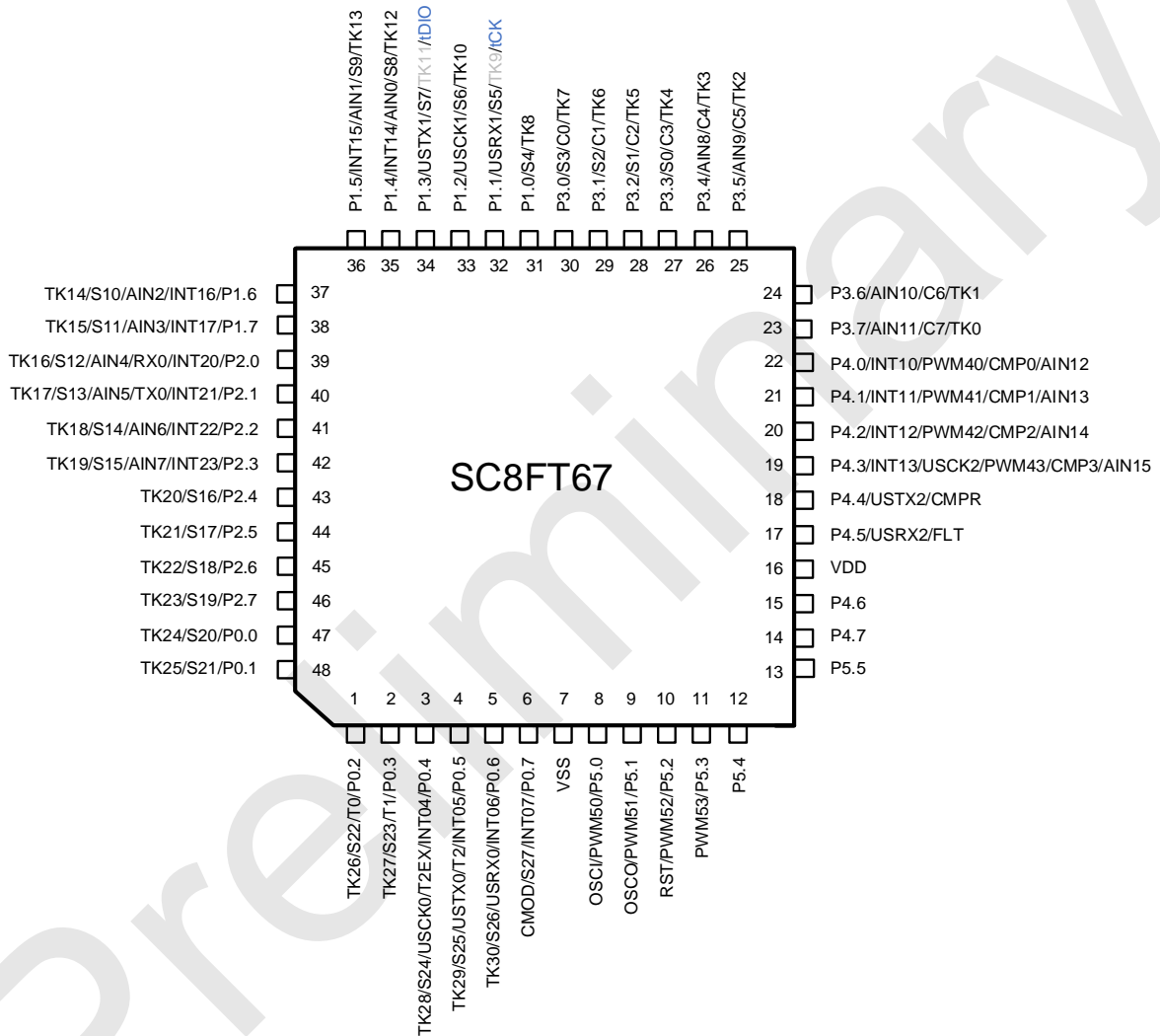
SC8FT67 管脚配置图
