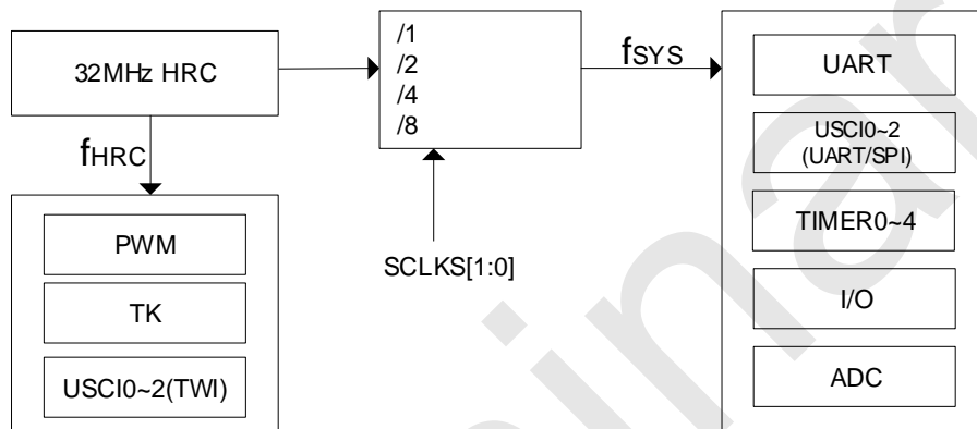
SC8FT67 内部时钟关系
