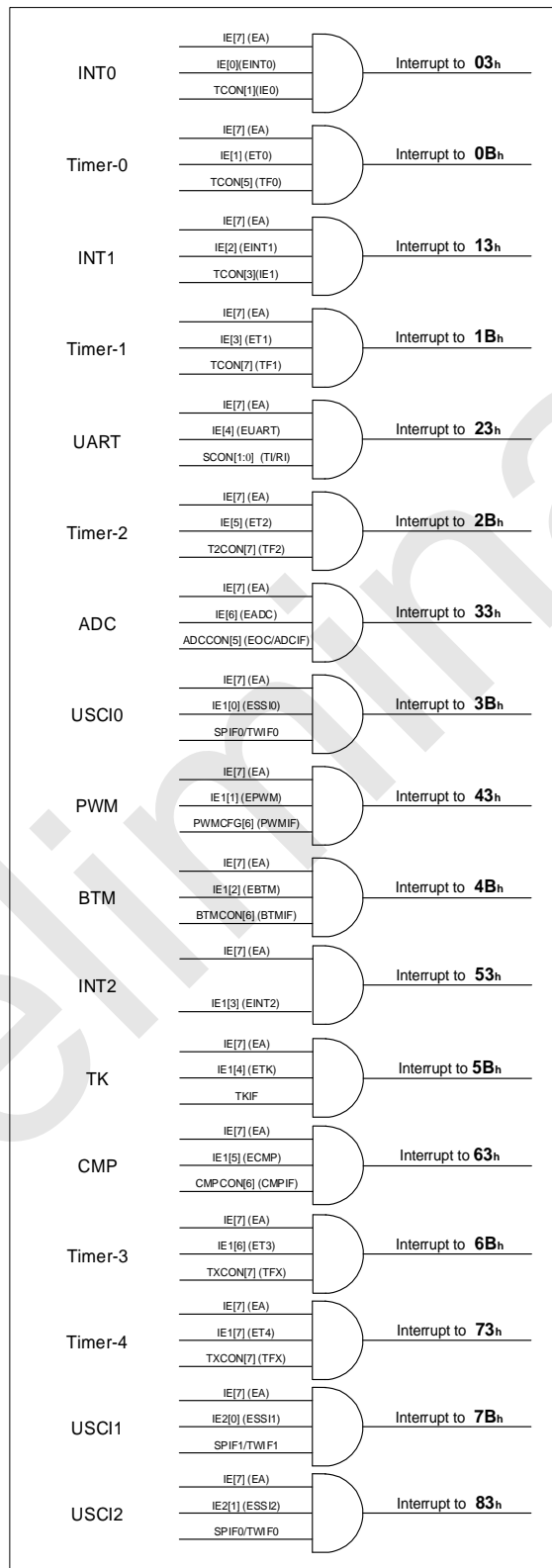
SC8FT67 中断结构和向量
