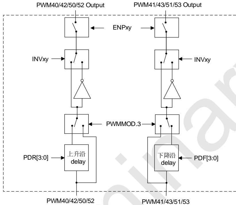
SC8FT67 PWM 互补模式框图
