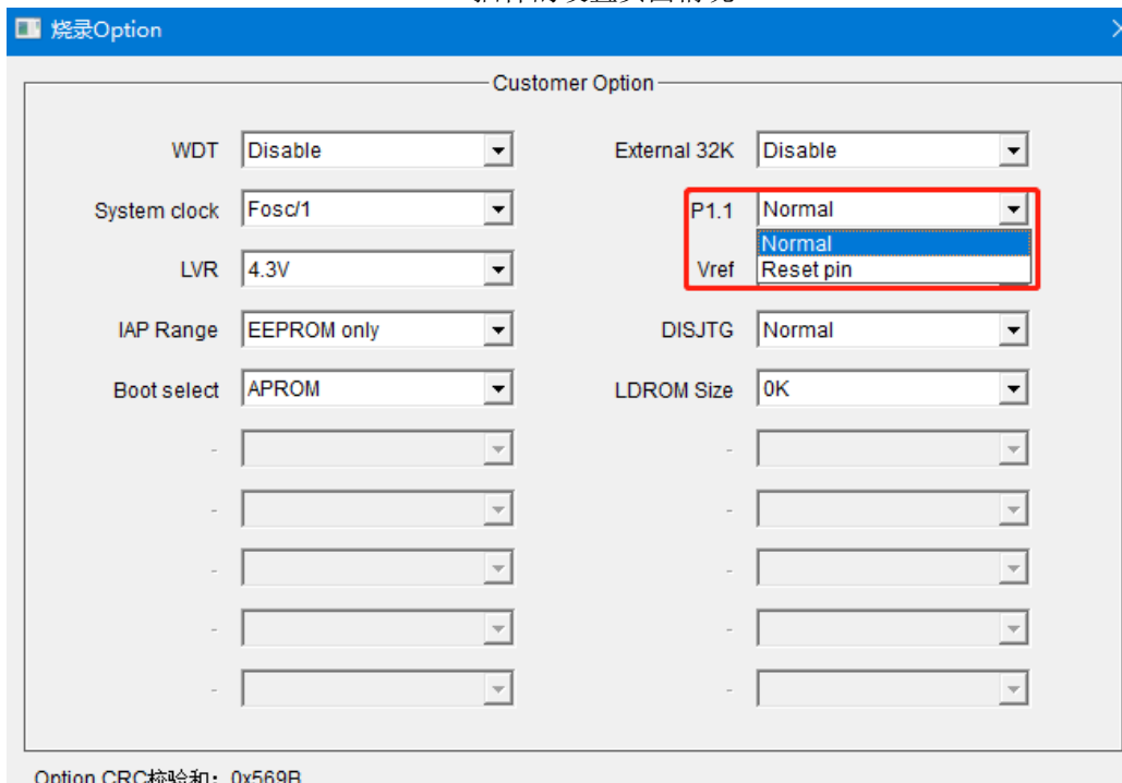
烧录上位机 SOC Programming Tool 的设置页面情况
