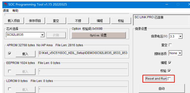
烧录上位机 SOC Programming Tool 设置页面
