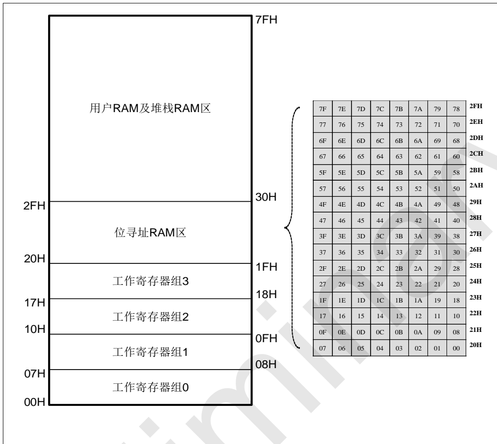
SRAM 结构图
