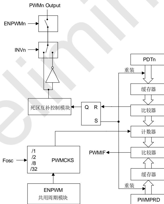
SC92F74AX PWM 结构框图
