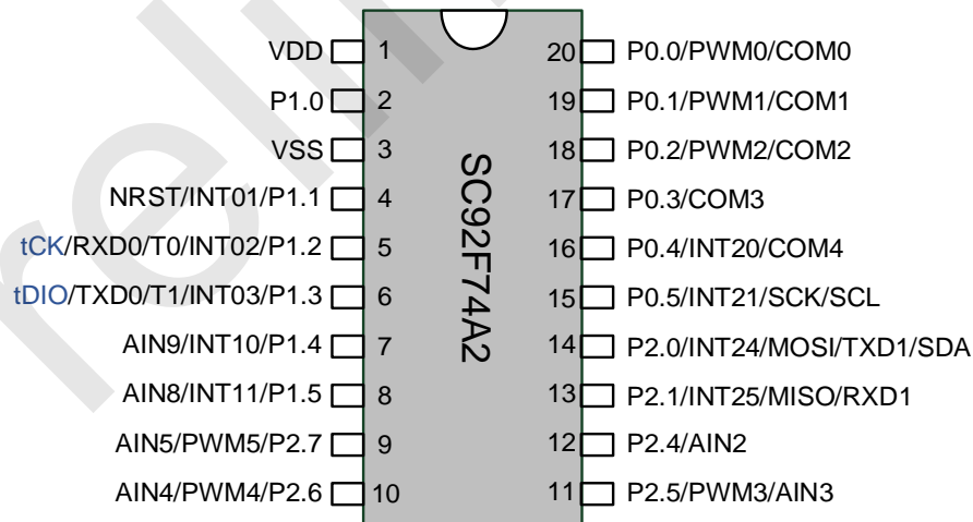
SC92F74A2 管脚配置图
