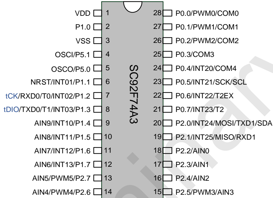
SC92F74A3 管脚配置图
