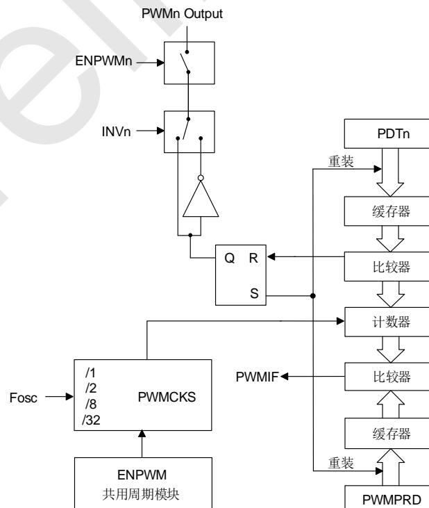
SC92F74AX PWM 独立模式框图
