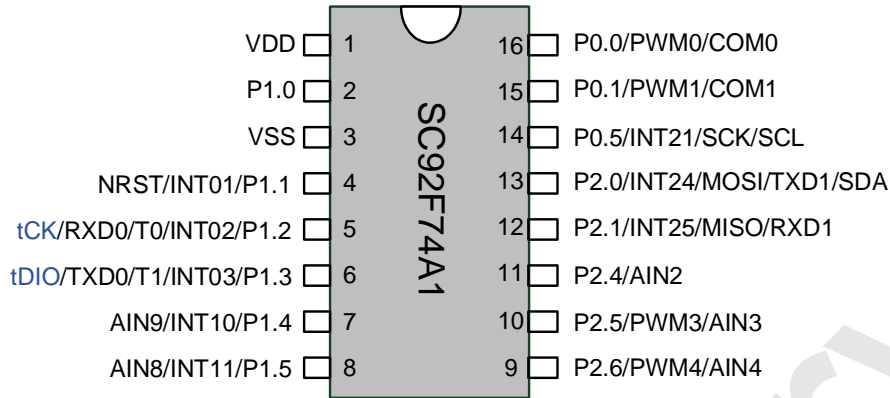
SC92F74A1 管脚配置图
