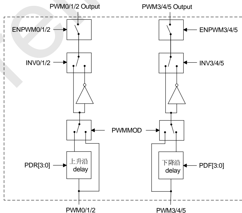
SC92F74AX PWM 互补模式框图
