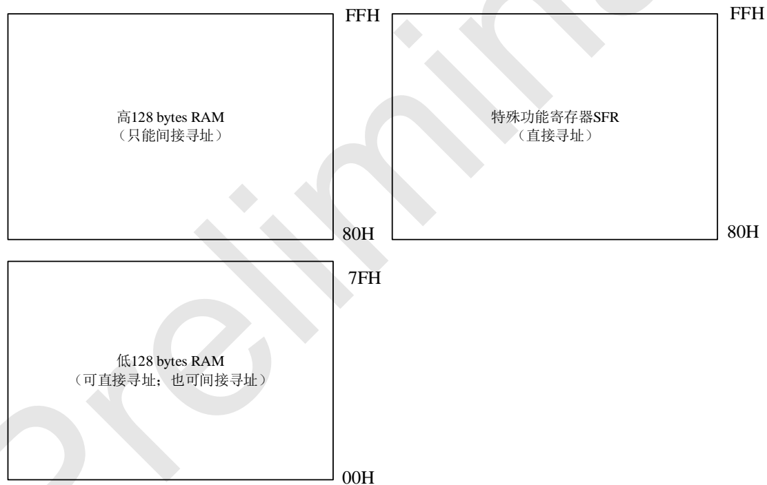
内部 256 bytes RAM 结构图
