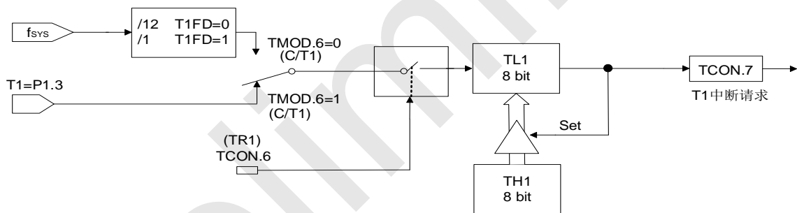
定时器/计数器工作模式 2: 自动重载的 8 位定时器/计数器
