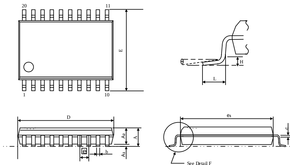
TSSOP20L 外形尺寸
