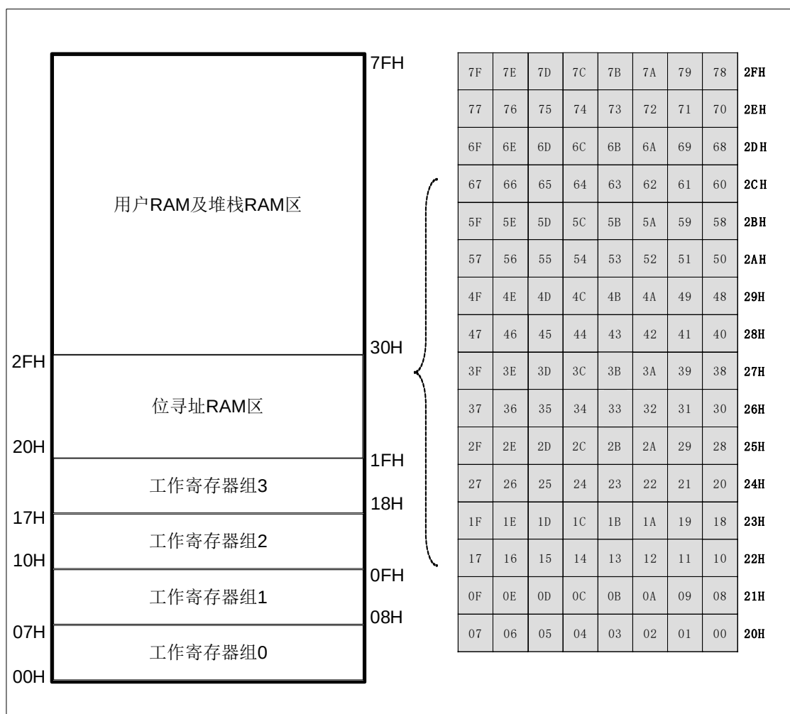
SRAM 结构图
