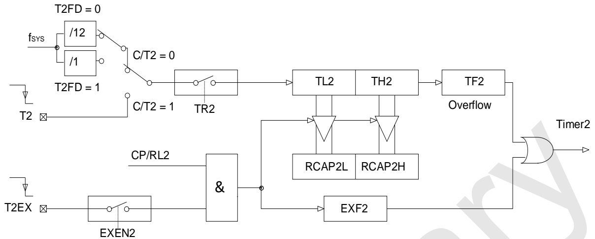
模式 0: 16 位捕获
