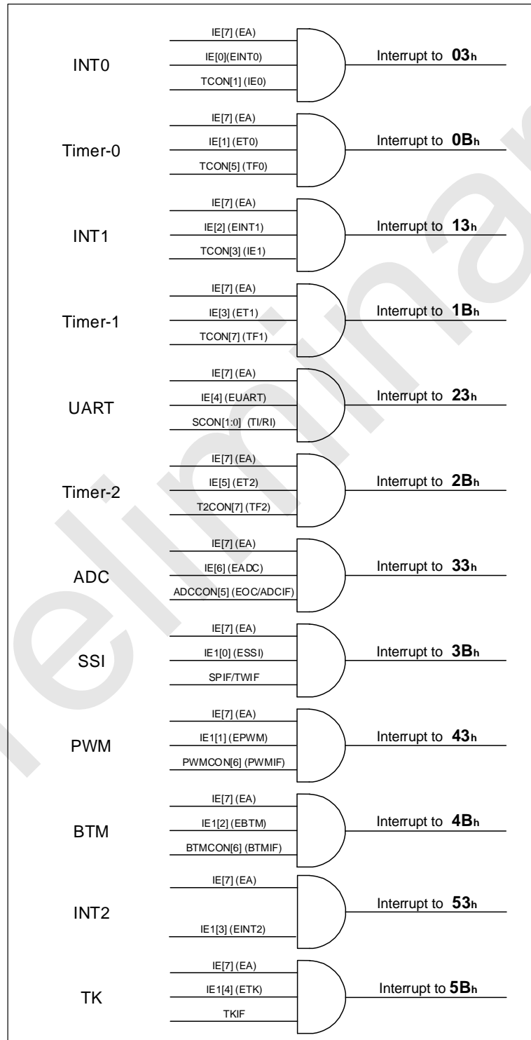
SC92F836XB 中断结构和向量
