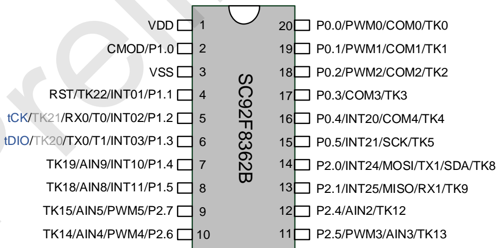
SC92F8362B 管脚配置图
