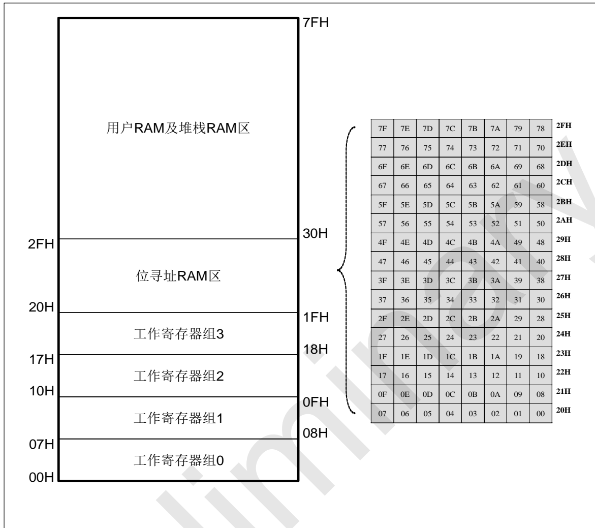
SRAM 结构图
