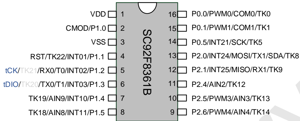
SC92F8361B 管脚配置图
