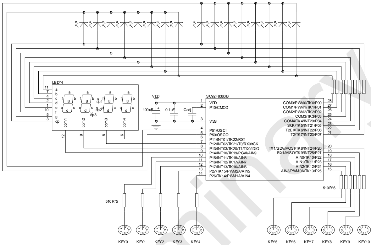
SC92F8363B Touch Key 应用电路图
