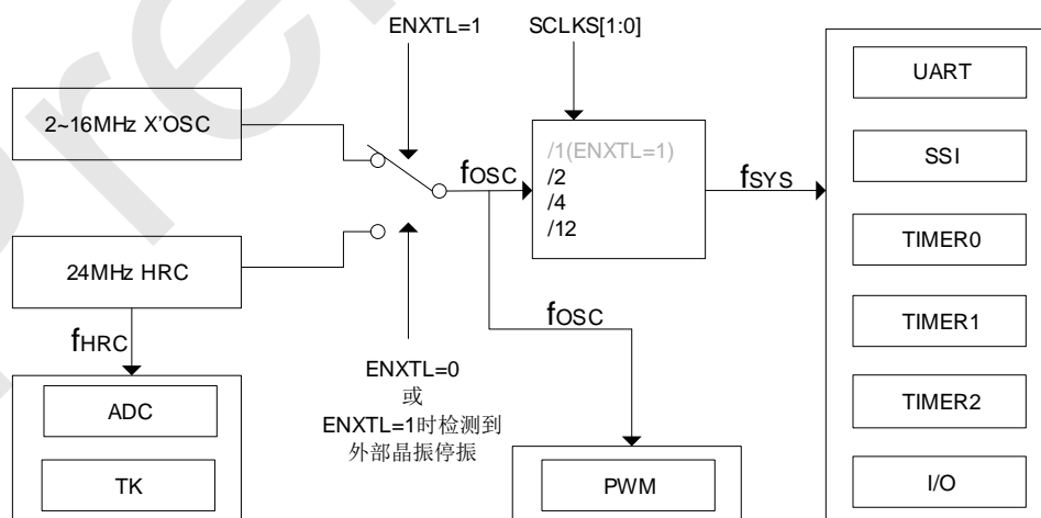
SC92F836XB 内部时钟关系
