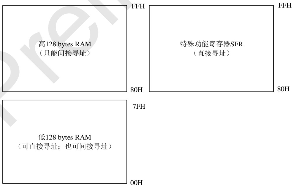
内部 256 bytes RAM 结构图
