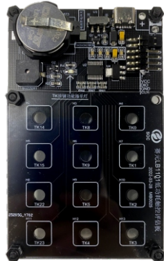
Lb1101开发板
