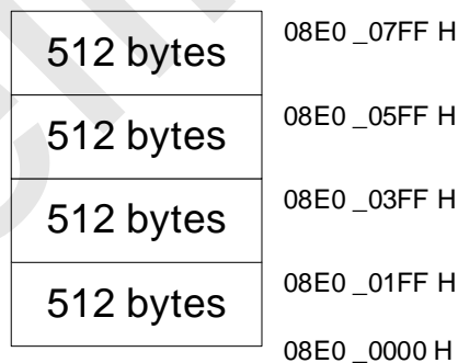
SC32F15G EEPROM Sector 分区示意
