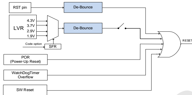
SC32F15G 复位电路图
