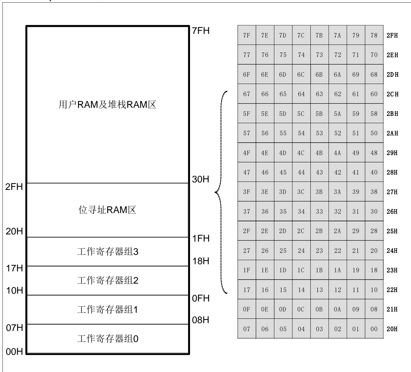
SRAM 结构图
