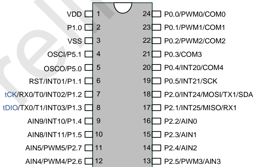
SSOP24 管脚配置图
