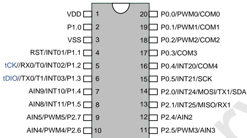
SOP20/TSSOP20 管脚配置图
