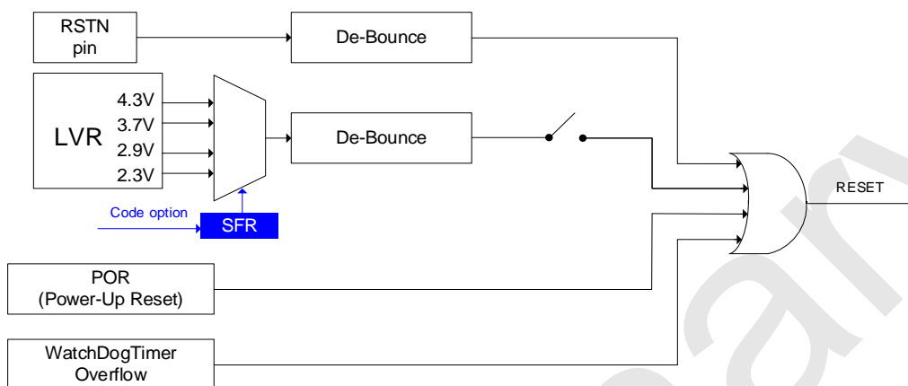
SC92F741XB 复位电路图
