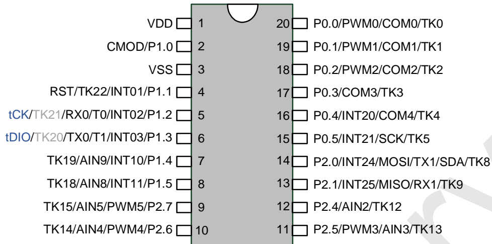
SOP20/TSSOP20 管脚配置图
