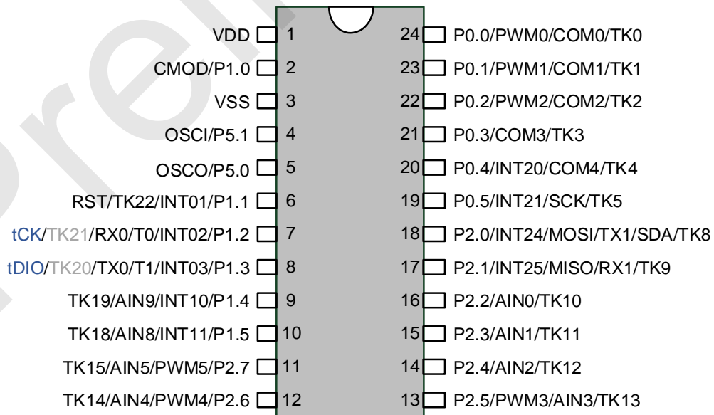
SSOP24 管脚配置图
