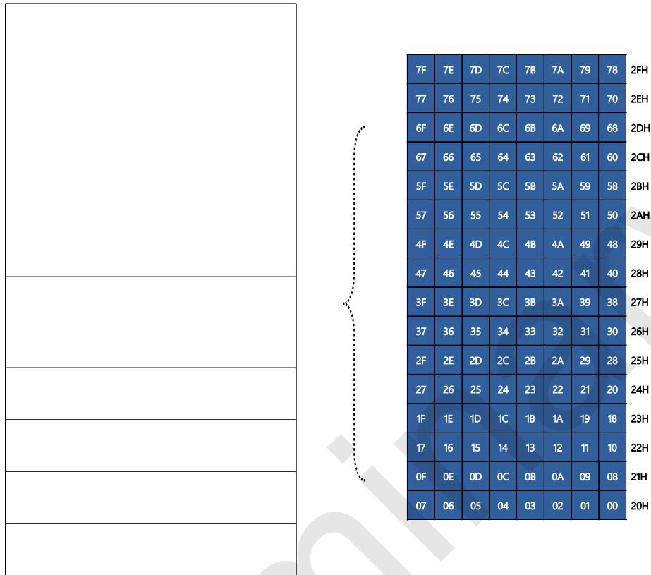
SRAM 结构图
