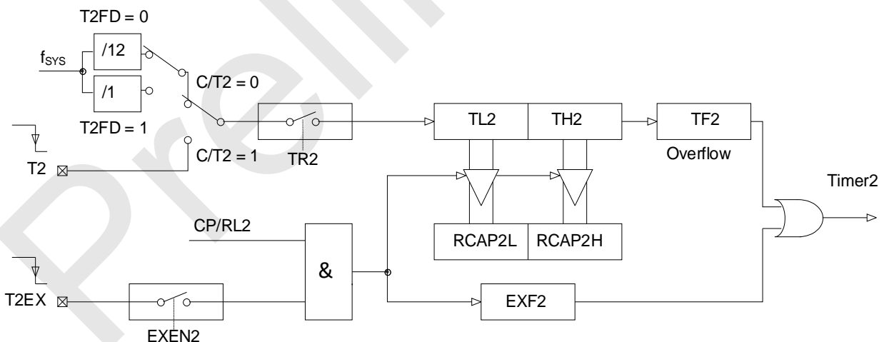
模式 0: 16 位捕获
