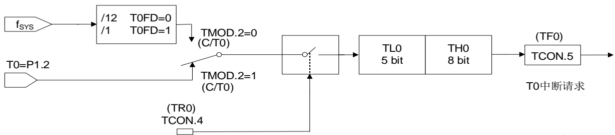
定时器/计数器工作模式 0: 13 位定时器/计数器
