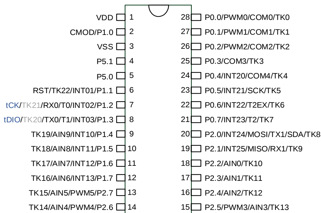
SC92F8483 管脚配置图
