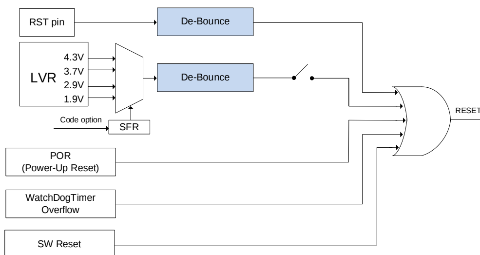
SC92F848X 复位电路图
