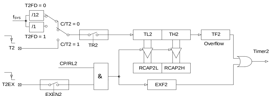
模式 0: 16 位捕获
