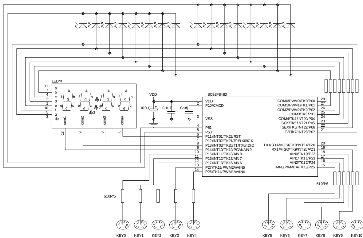
SC92F8483 Touch Key 应用电路图
