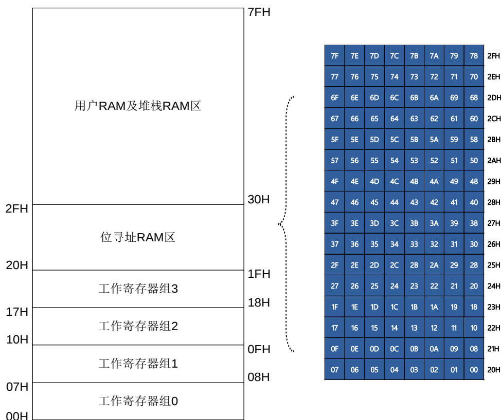
SRAM 结构图
