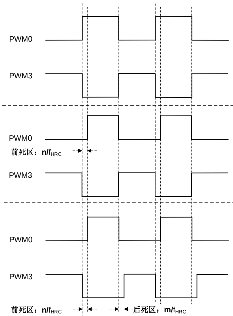
PWM 死区输出波形
