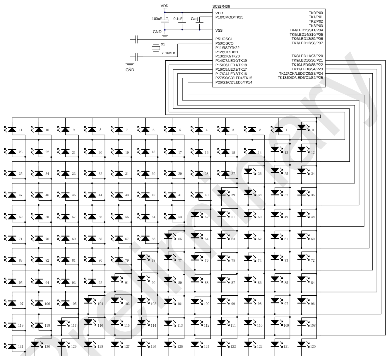
SC92R436 Touch Key 应用电路图
