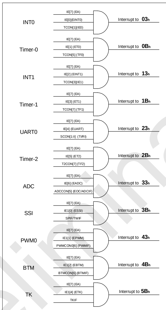
SC92R436 中断结构和向量
