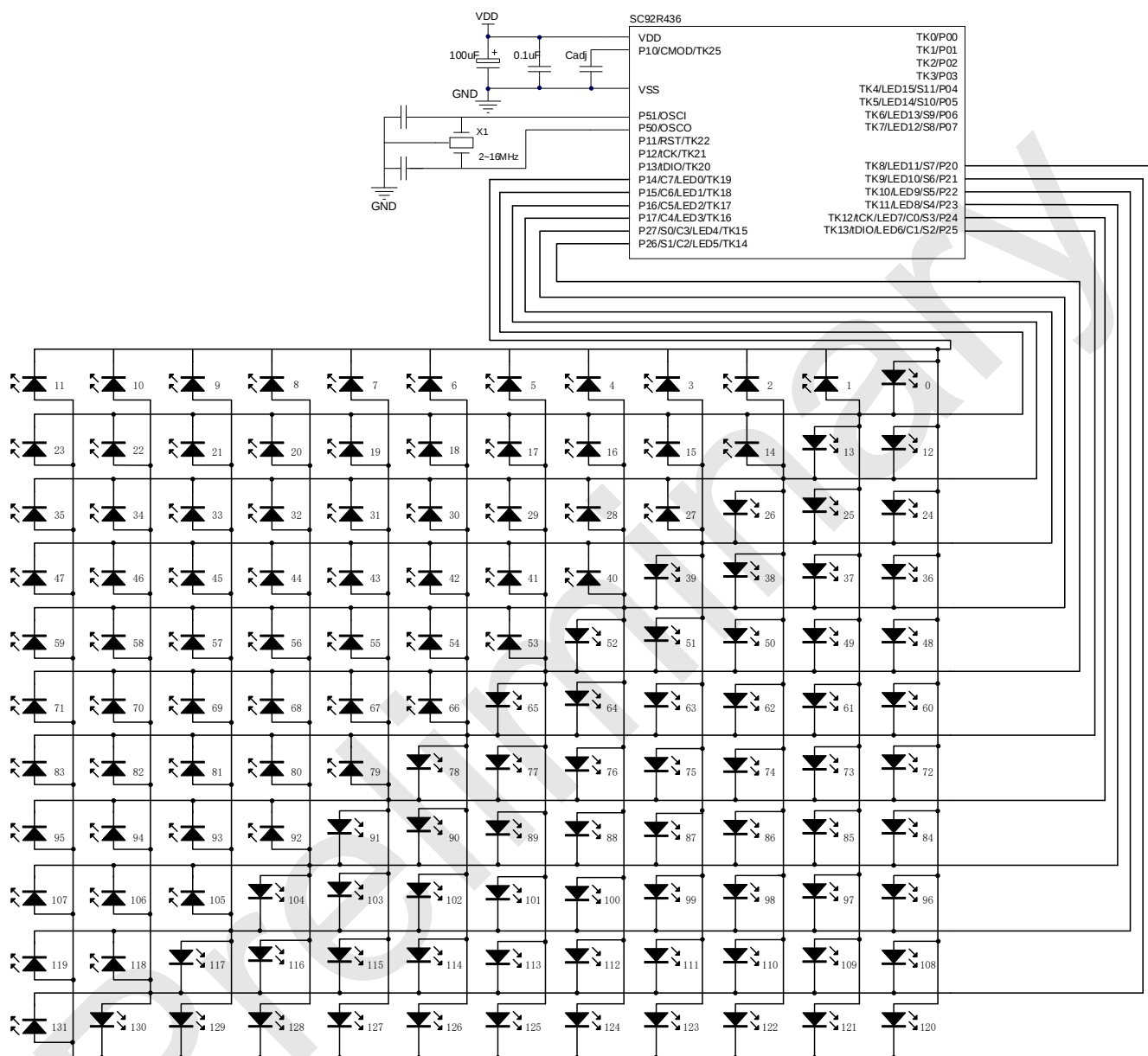
SC92R436 正反推模式 LED 应用电路图
