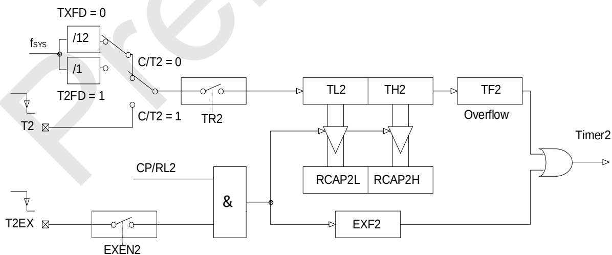
模式 0: 16 位捕获
