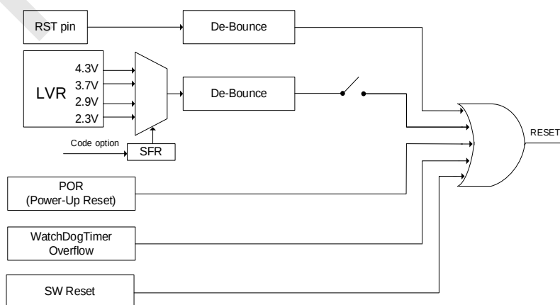
SC92R436 复位电路图
