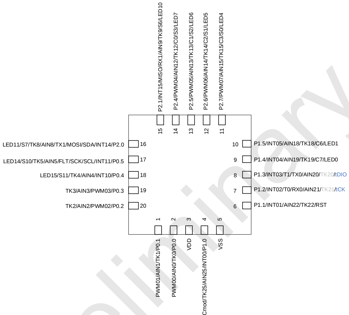
SC92R436 管脚配置图 适用于 QFN20 封装
