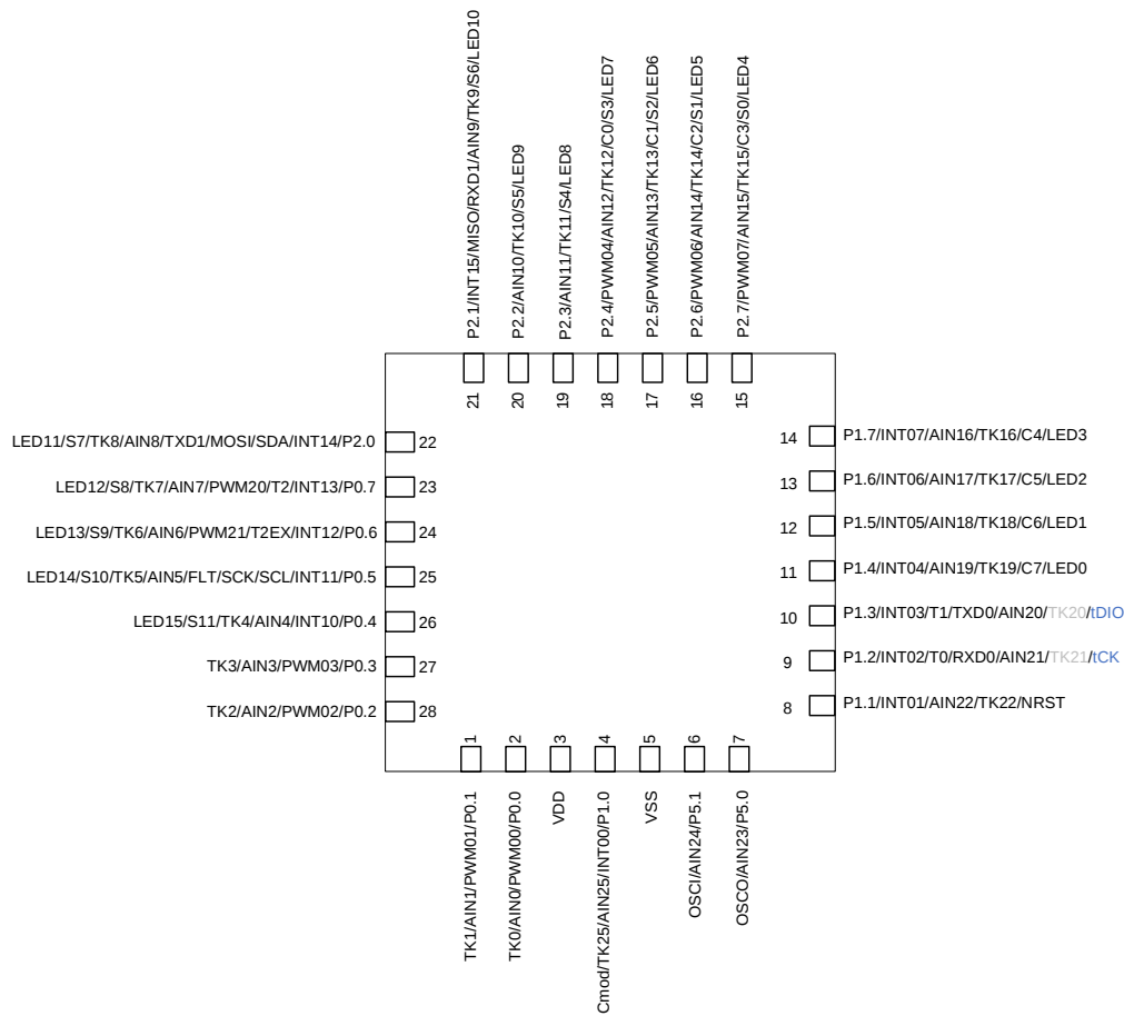
SC92R436 管脚配置图
