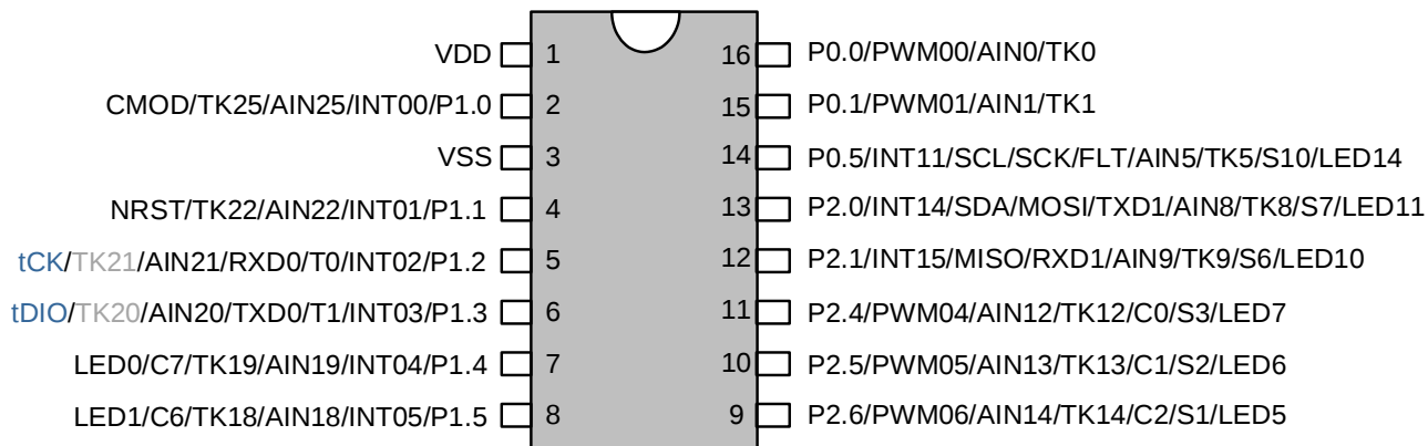
SC92R436 管脚配置图
