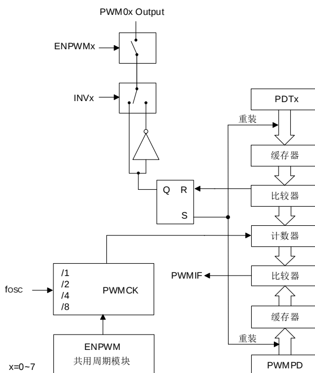
SC92R436 PWM 独立模式框图
