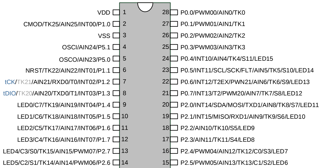
SC92R436 管脚配置图
