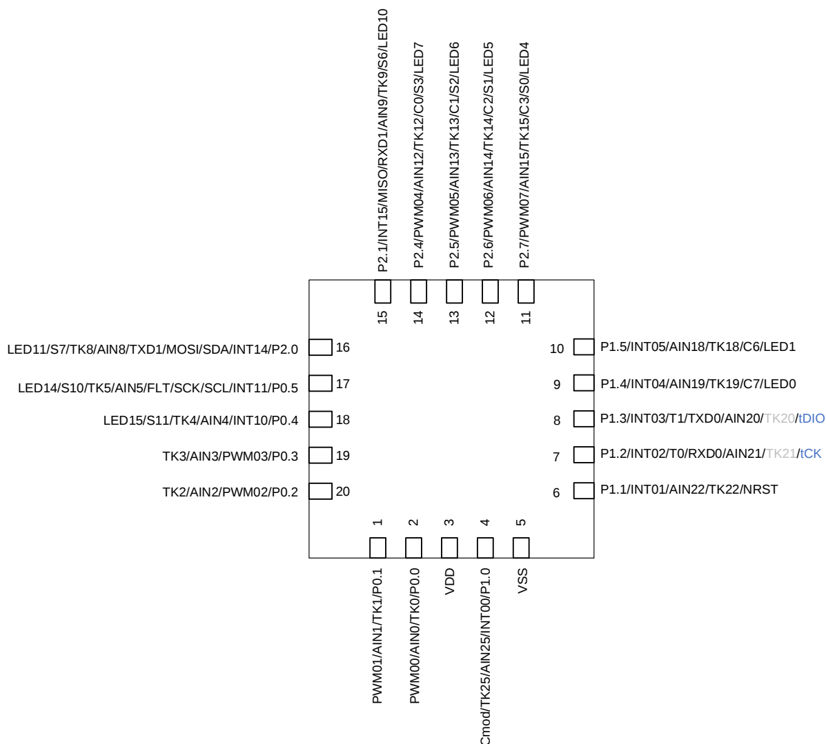
SC92R436 管脚配置图
