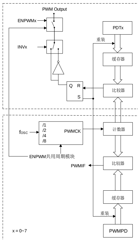
SC92R436 PWM 结构框图
