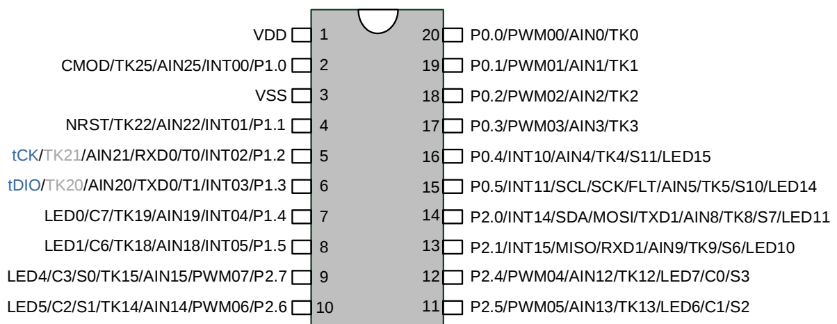
SC92R436 管脚配置图
