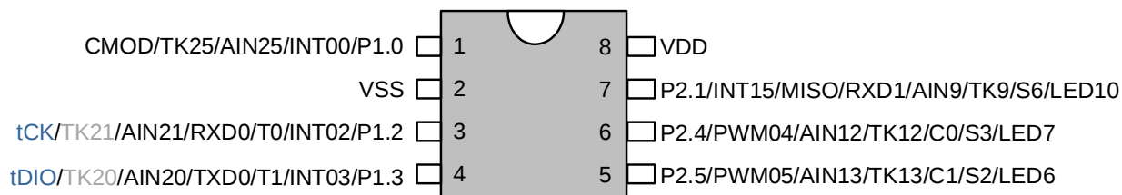
SC92R436 管脚配置图
