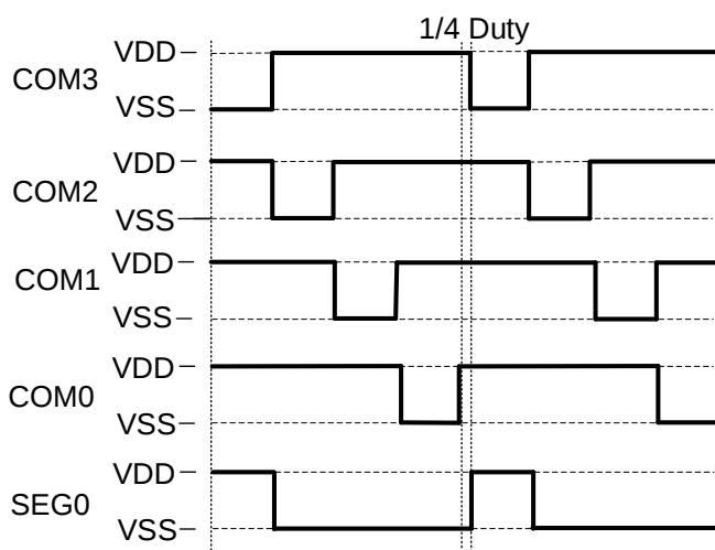
LED 应用中 COM 和 SEG 的波形图
