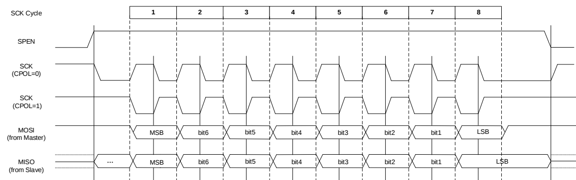
CPHA = 1 数据传输图
