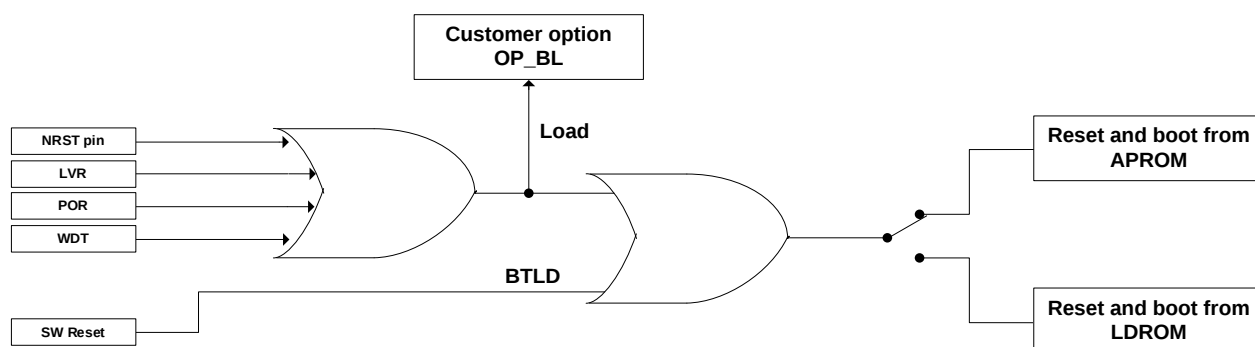
SC92R436 复位后启动区域切换示意图
