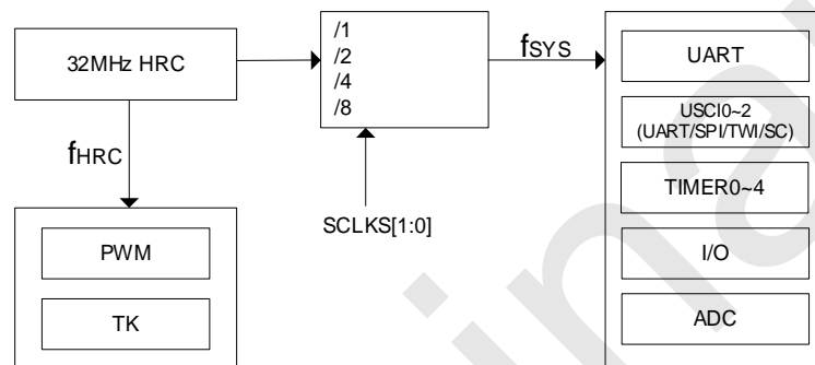
SC95F852X 内部时钟关系
