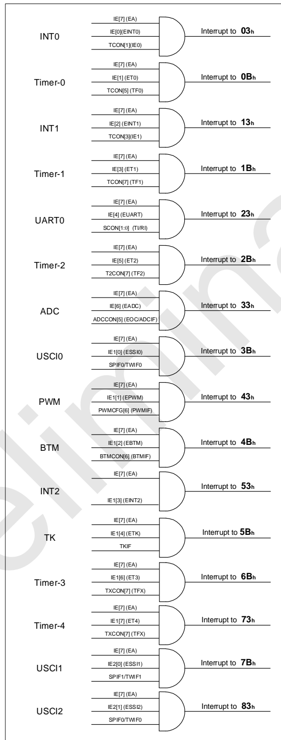
SC95F852X 中断结构和向量
