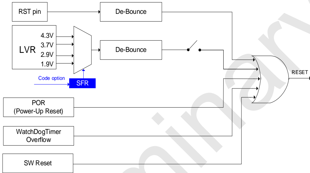
SC95F852X 复位电路图
