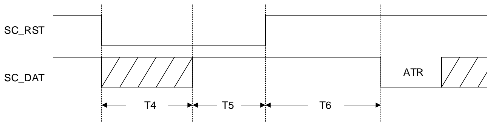
SC 暖复位时序
