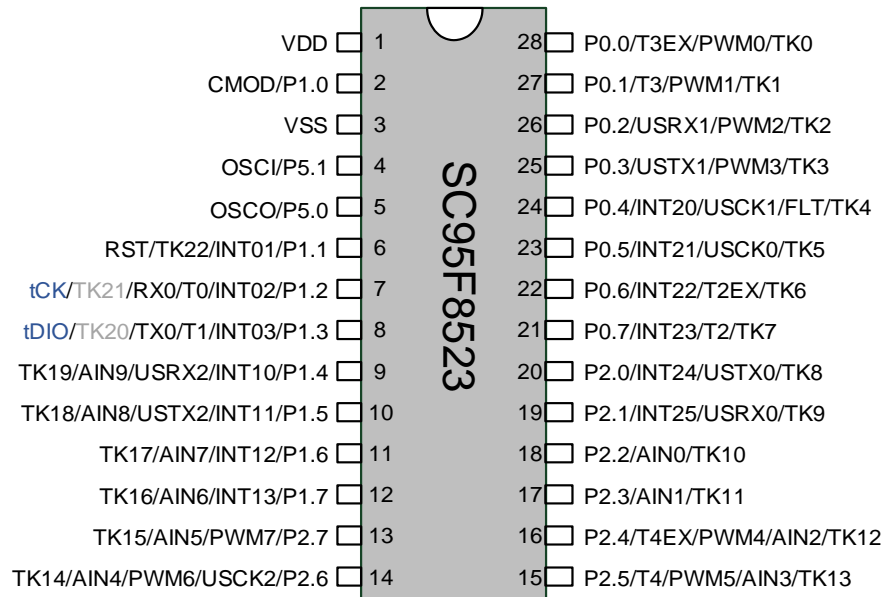
SC95F8523 管脚配置图
