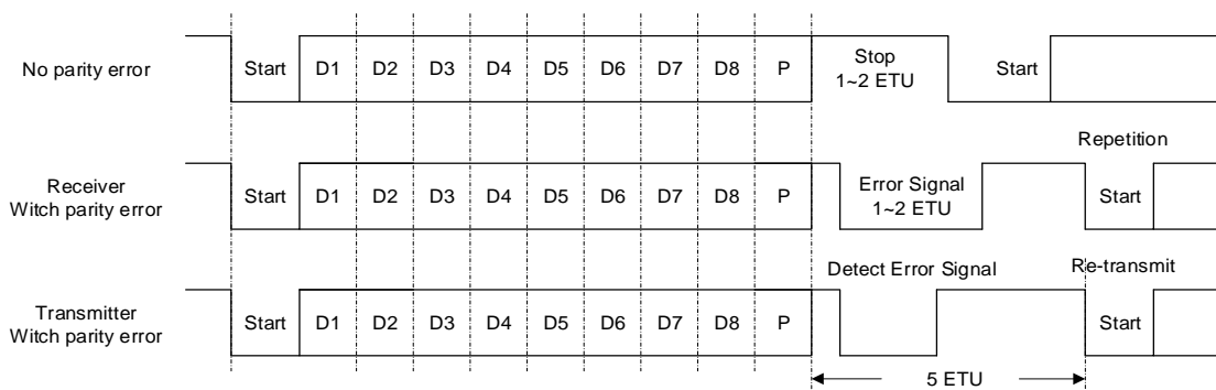
SC 错误信号
