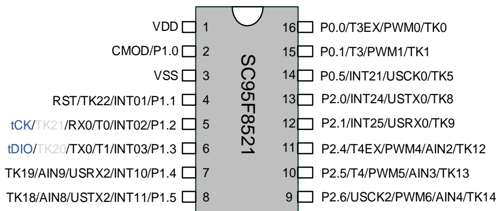
SC95F8521 管脚配置图
