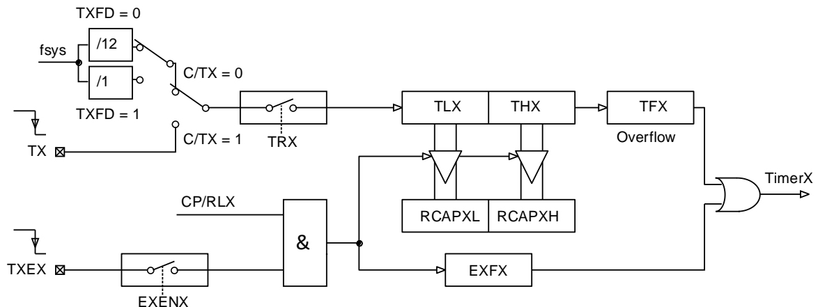
模式 0：16 位捕获
