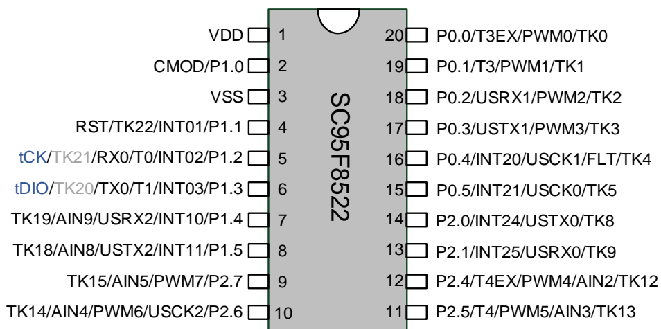
SC95F8522 管脚配置图
