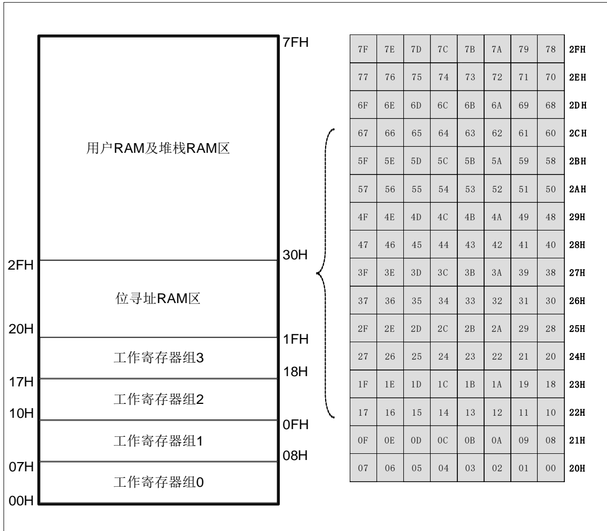
SRAM 结构图
