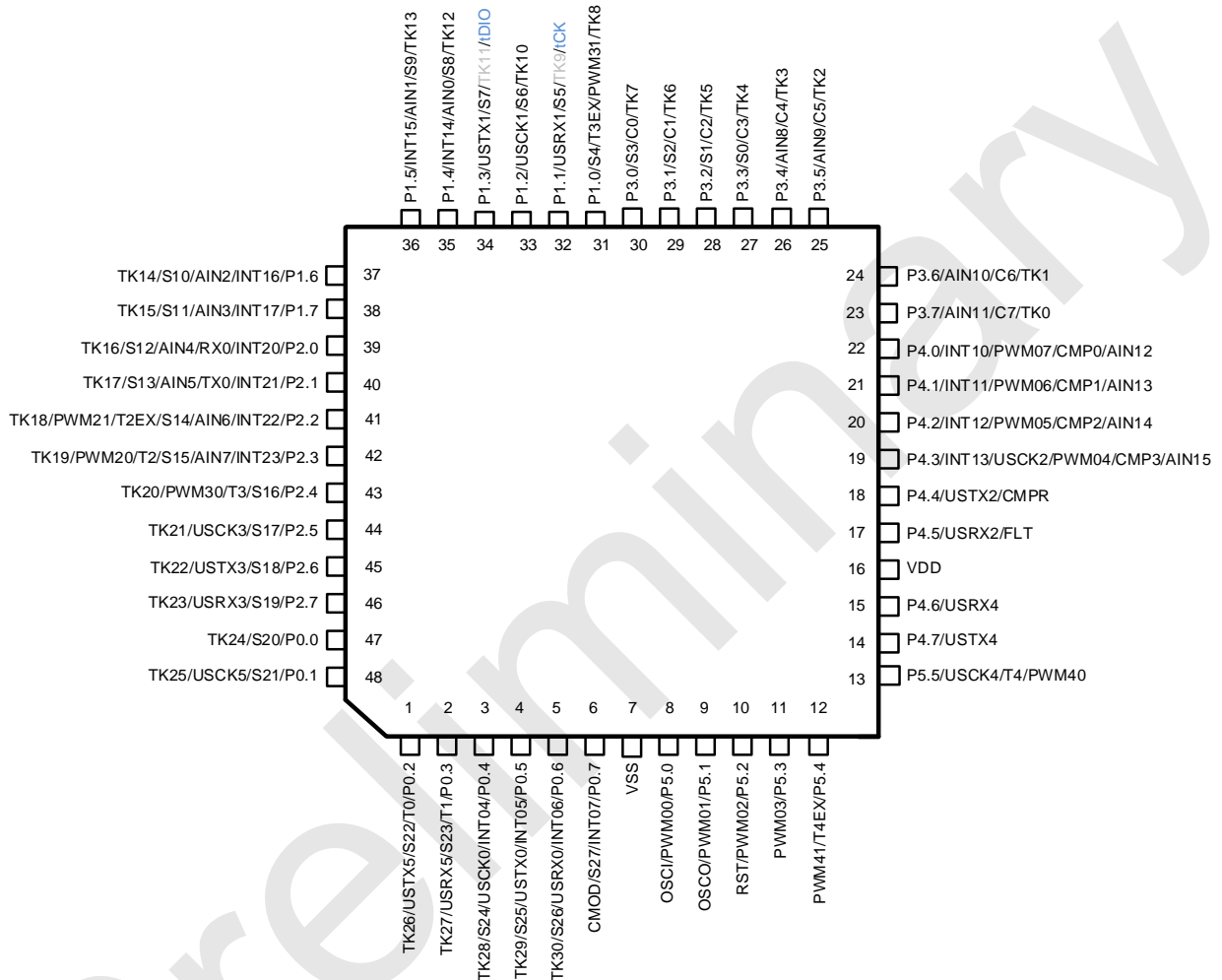
SC95F8617B 管脚配置图 适用于 LQFP48 封装
