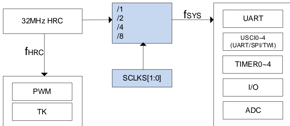
SC95F873X 内部时钟关系
