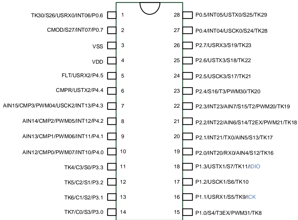
28PIN 管脚配置
