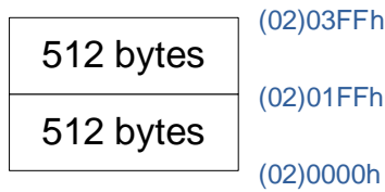
SC95F873X EEPROM Sector 分区示意
