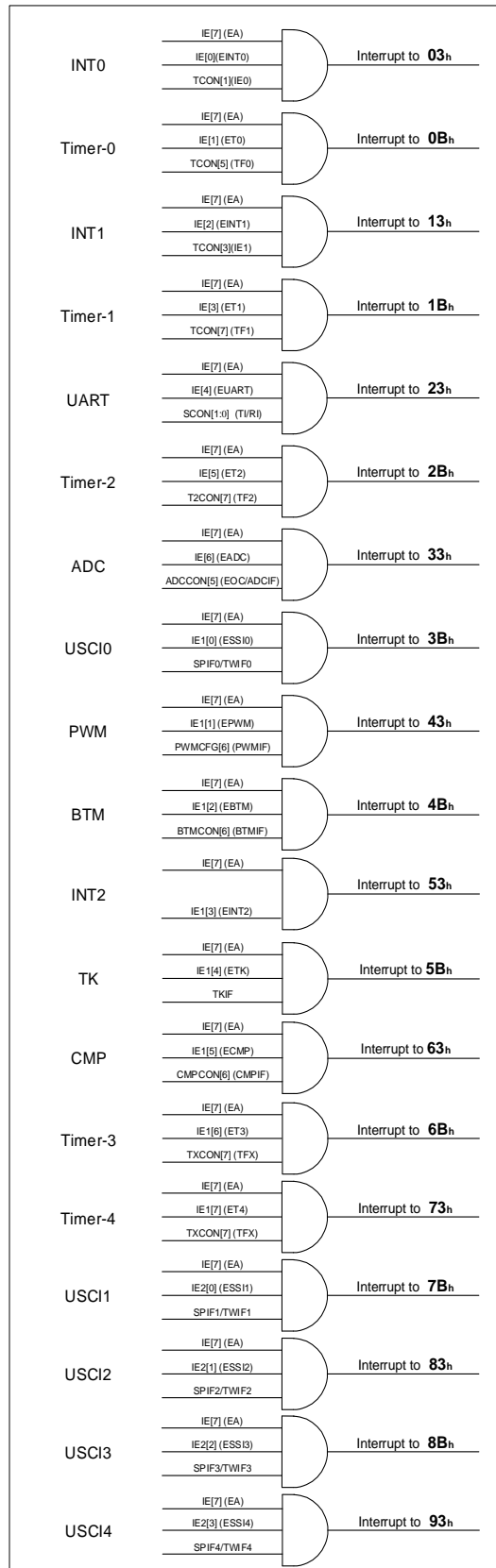
SC95F873X 中断结构和向量
