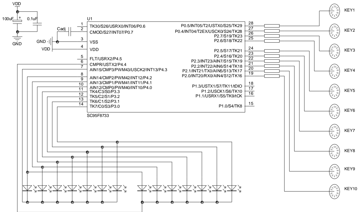
SC95F8733 Touch Key 应用电路图
