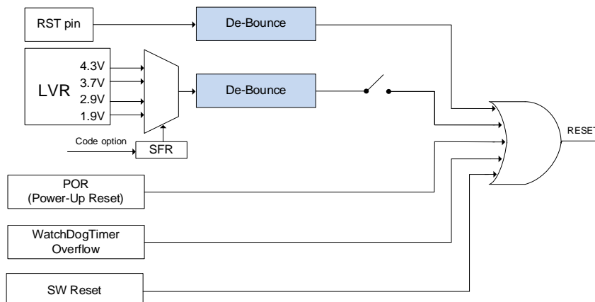
SC95F873X 复位电路图
