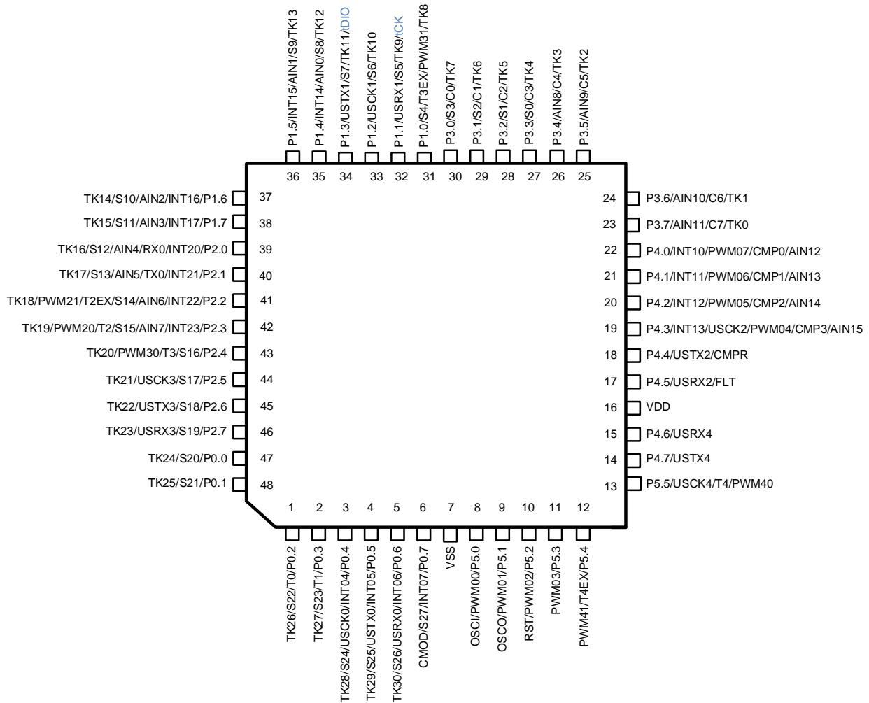
48PIN 管脚配置图
