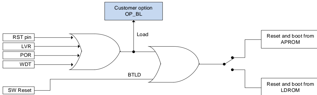
SC95F873X 复位后启动区域切换示意图
