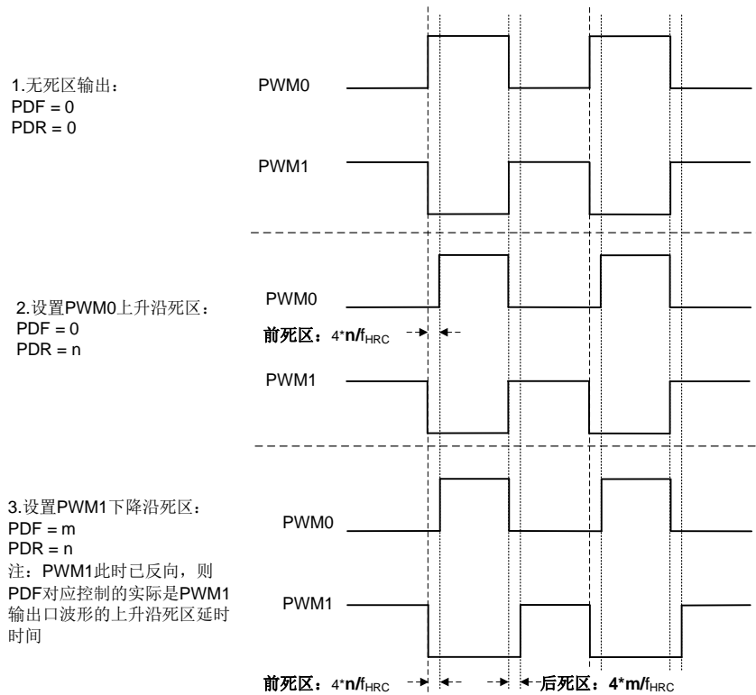
PWM0 死区输出波形
