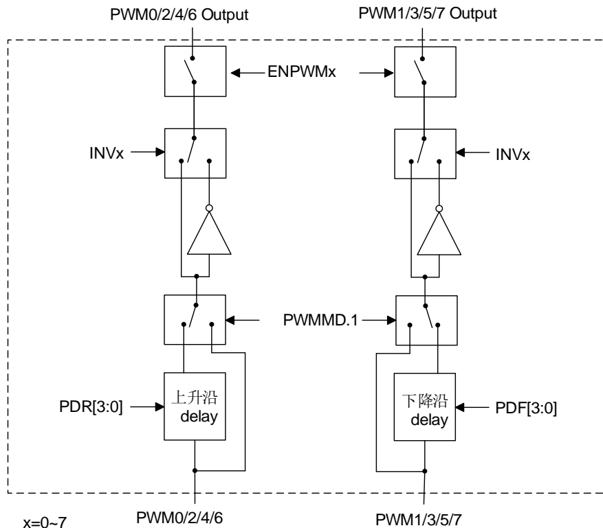
SC95F873X PWM 互补模式框图
