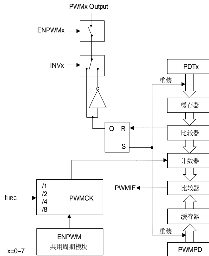
SC95F873X PWM 独立模式框图
