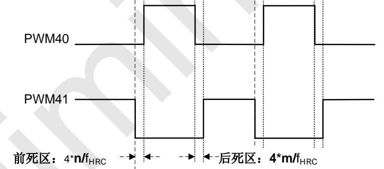
PWM1 死区输出波形
