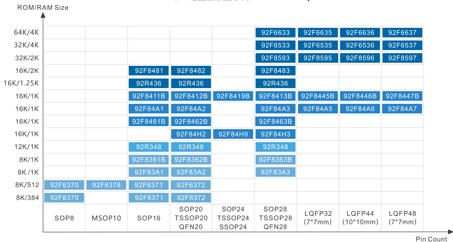
92F8/F6超值型触控系列MCU Roadmap
